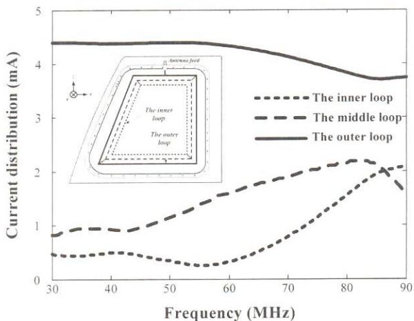
그림 7. 주파수에 따른 전류 분포 Fig. 7. Current distribution vs. frequency.
