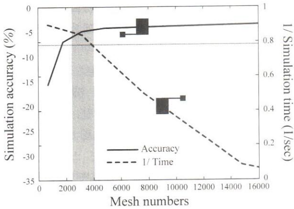
그림 3. 동체 mesh수에 따른 EM 시뮬레이션 정확도 및 해석 시간 Fig. 3. Accuracy and simulation time vs. aircraft mesh numbers.
