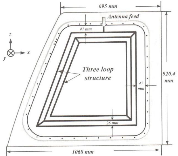
그림 4. 최적화된 안테나 형상 Fig. 4. The optimized on-glass antenna structure.
